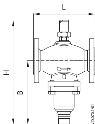
VFQ Ду15-125
